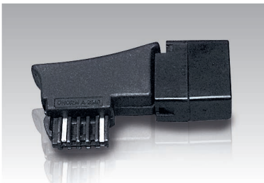
Anschlussadapter TST-Stecker – RJ11-Buchse 4-adrig verschalteter Anschlussadapter für Telefone und Zusatzgeräte Connector adapter TST plug – RJ11 socket 4-core fully-wired connector adapter for telephones and accessories
