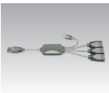
USB 2.0 HUB 3+1 Mini USB B Port, flexibel Kompakter USB 2.0 HUB mit 3 flexiblen USB A Buchsen (Kupplungen) und 1 flexiblen Mini USB B Stecker (5pin). Ideal für den direkten Anschluss der Geräte mit Mini USB B Stecker, z.B. MP3, Digital Kamera etc. • 1 Upstream und 4 Downstream USB ports
